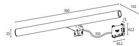
Cotas Técnicas / Technical Dimensions
