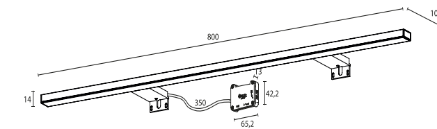
Cotas Técnicas / Technical Dimensions
